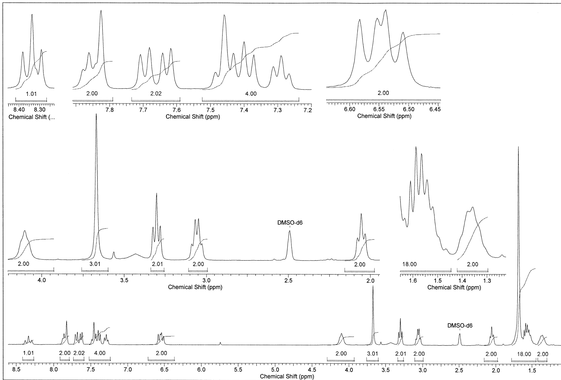
^1\text{H} NMR ( \text{DMSO-}d_6 , 300 MHz)
