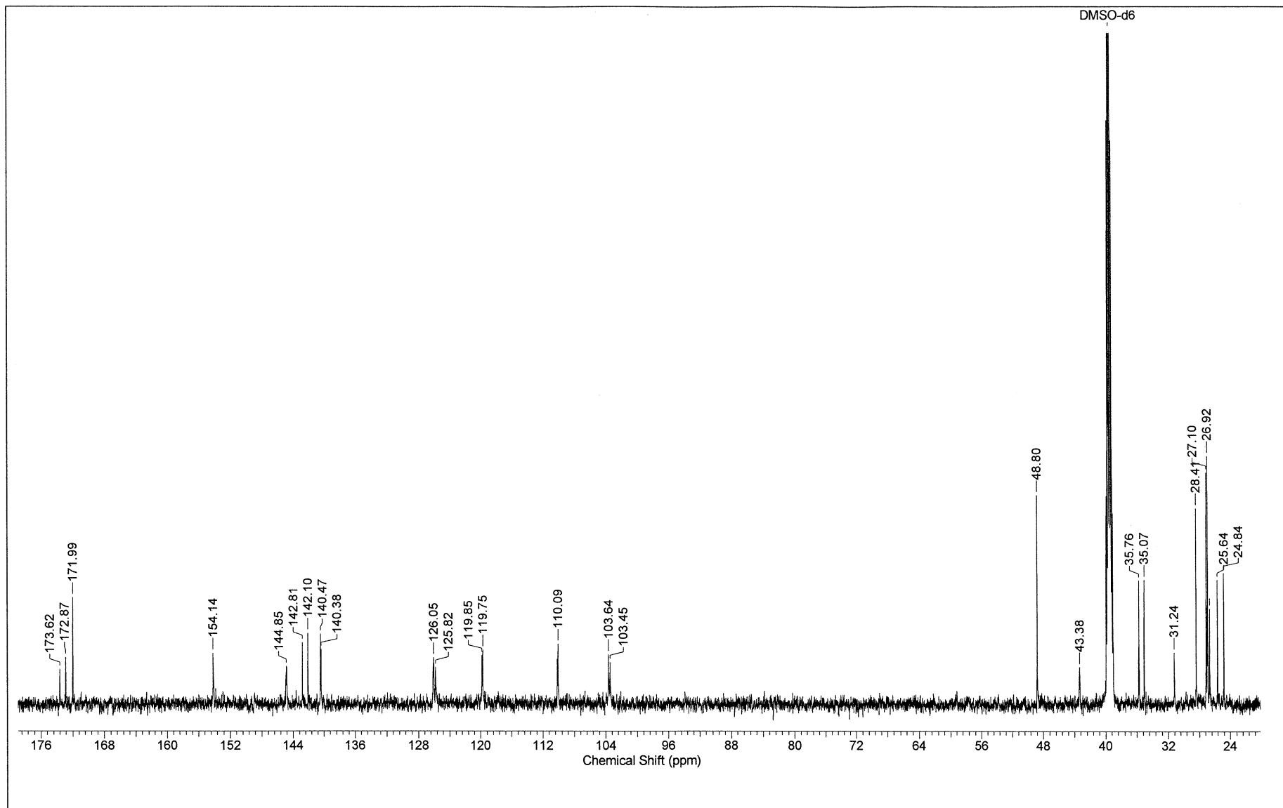
13 C NMR (DMSO-d 6 , 150 MHz)
