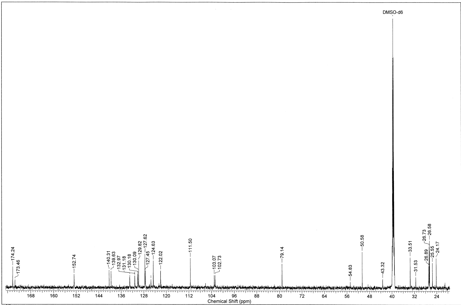
13 C NMR (DMSO-d 6 , 150 MHz)
