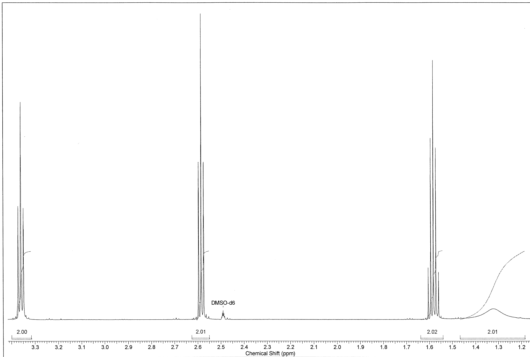
^1\text{H} NMR (DMSO- d 6 , 600 MHz)
